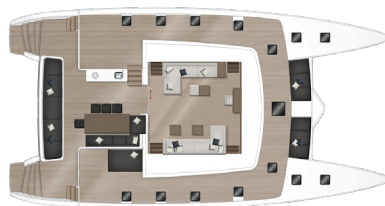
Carré et cockpit avec cuisine latérale
