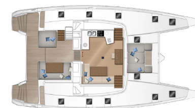
Carré et cockpit
