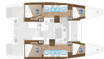
Version 4 cabines, 4 salles de bain
