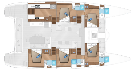
Version 5 cabines - cuisine latérale
