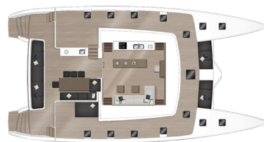
Carré et cockpit avec cuisine latérale
